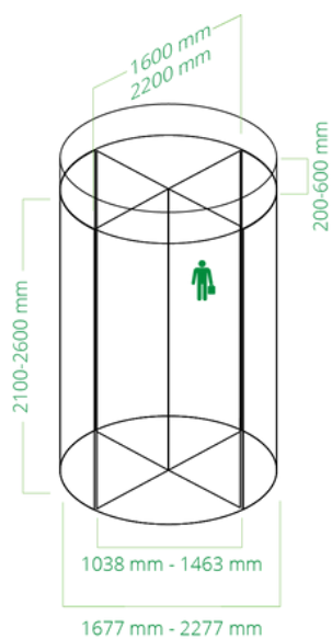
BEVEILIGDE ZIJDE
