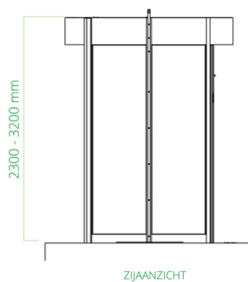
ZIJAAANZICHT
