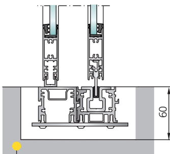
Doorlopende in de vloer ingewerkte vloerrail (verhoogt de veiligheid en de stabiliteit)
