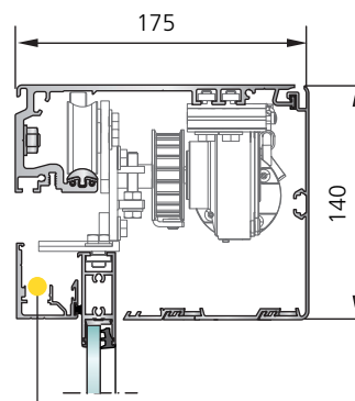
SL 35-S Afkasting rond de aandrijving hoogte 140 mm zonder zijprofiel (verkrijgbaar met draagprofiel)
