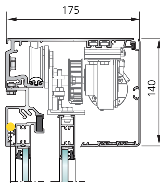
SL 35-S Afkasting rond de aandrijving hoogte 140 mm met zijprofiel (verkrijgbaar met draagprofiel)
