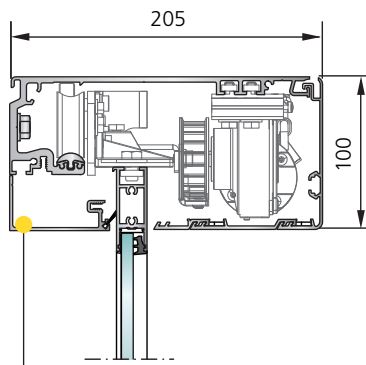
SL 35-C Afkasting rond de aandrijving hoogte 100 m zonder zijprofiel
