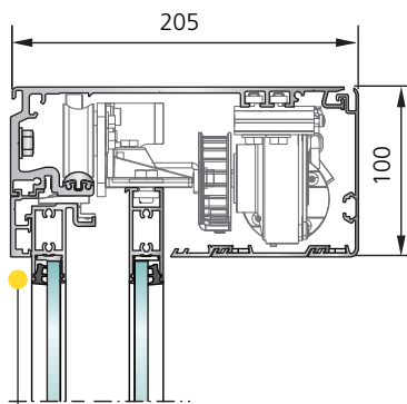
SL 35-C Afkasting rond de aandrijving hoogte 100 mm met zijprofiel
