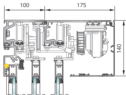
SL 35-T Afkasting rond de telescopische aandrijving hoogte 140 mm met zijprofiel (verkrijgbaar met draagprofiel)
