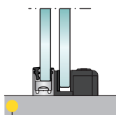
Glijvoet met zijdelingse vastpunteigleiding op de grond
