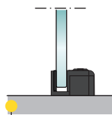
Glijvoet met zijdelingse vastpunteigleiding op de grond
