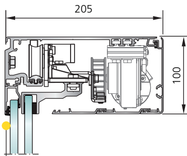
SL 35-C Afkasting rond de aandrijving : hoogte 100 mm met zijprofiel
