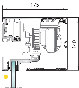
SL 35-C Afkasting rond de aandrijving : hoogte 140 mm zonder zijprofiel met borstelafdichting
