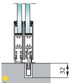
Geïntegreerde vloerrail in roestvrij staal over de volledige deurbreedte (verhoogt de bescherming tegen inbraak en de deurstabiliteit)
