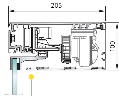
SL 35-C Afkasting rond de aandrijving : hoogte 100 mms zonder zijprofiel
