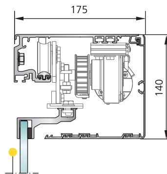
SL 35-C Afkasting rond de aandrijving : hoogte 140 mm zonder zijprofiel
