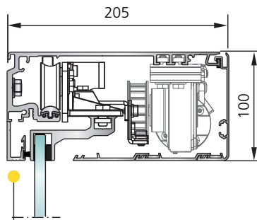
SL 35-C Afkasting rond de aandrijving : hoogte 100 mm zonder zijprofiel met borstelafdichting
