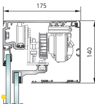
SL 35-C Afkasting rond de aandrijving : hoogte 140 mm met zijprofiel
