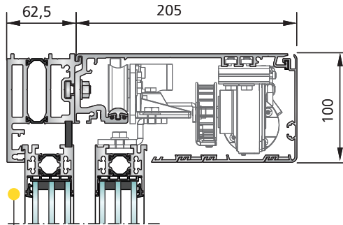
SL 35-C Afkasting rond de aandrijving hoogte 100 mm met zijpaneel en montageprofiel
