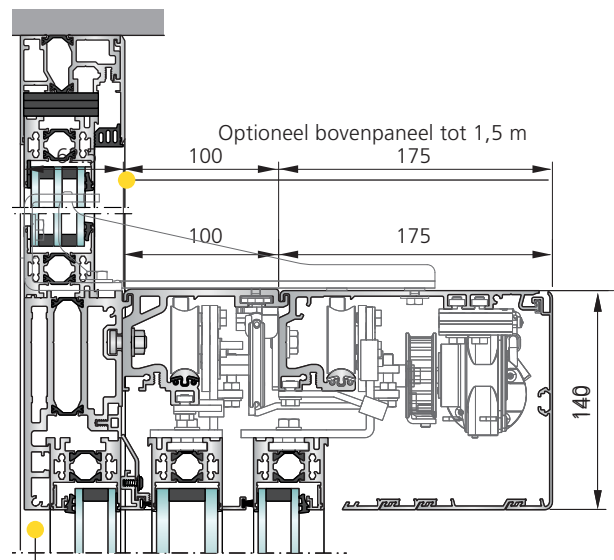
SL 35-T Afkasting rond de aandrijving hoogte 140 mm met zijpaneel en montageprofiel
