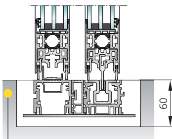
In de vloer ingewerkte rail (verhoogt de veiligheid en de stabiliteit), vloerrail met afwatering in optie
