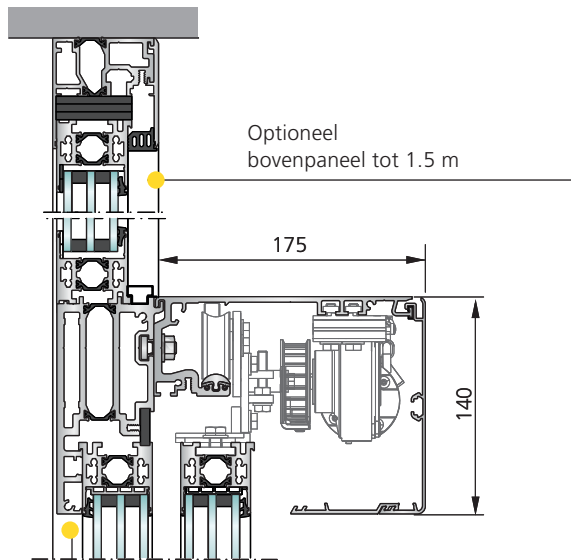
SL 35-S / SL 45-S Afkasting rond de aandrijving hoogte 140 mm met zijpaneel en montageprofiel
