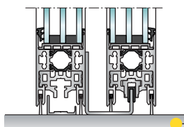
Glijvoet met vast vastpunt-geleiding
