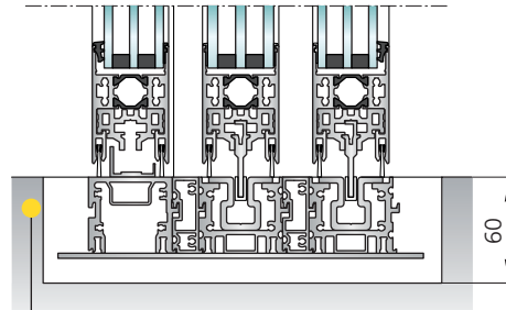
Telescopische vloerrail, vloerrail met afwatering in optie
