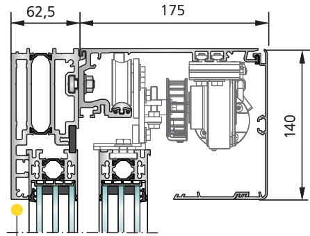
SL 35-S / SL 45-S Afkasting rond de aandrijving hoogte 140 mm met zijpaneel en montageprofiel
